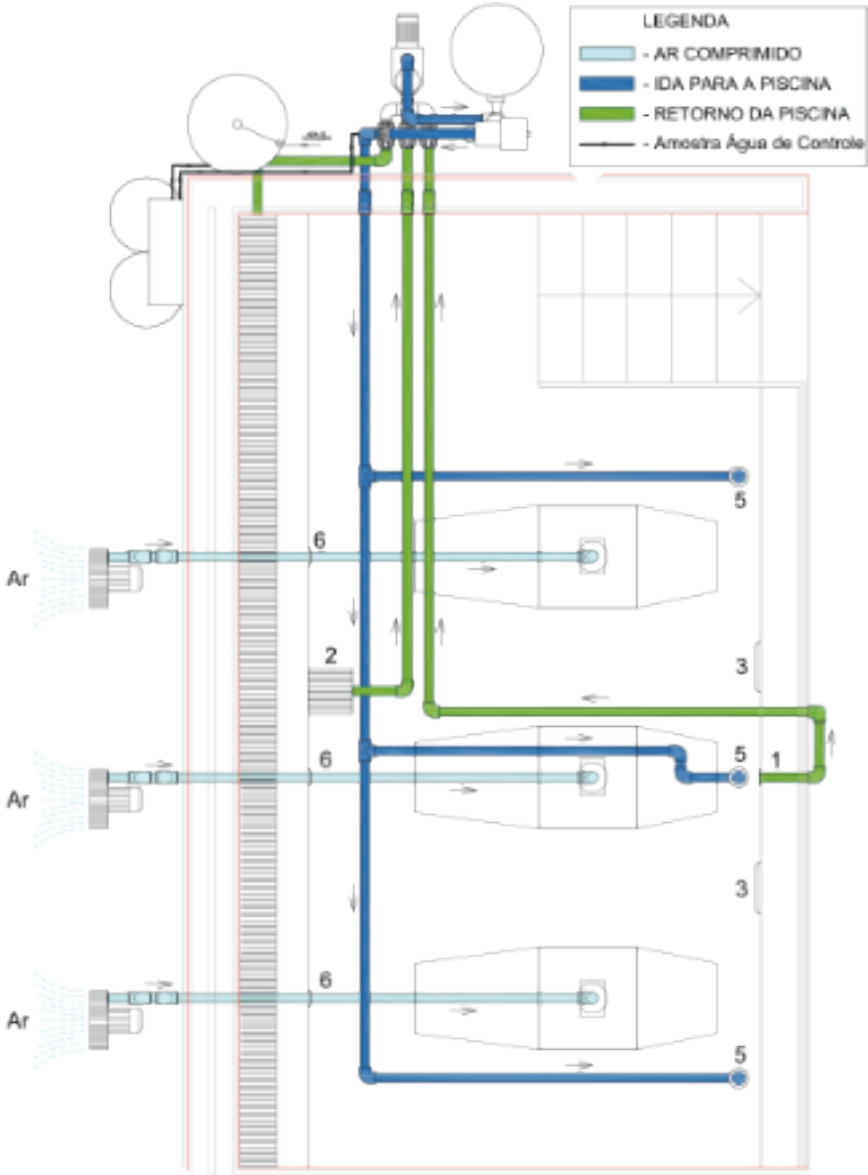
Legenda: esquema de organização da casa de máquinas.
